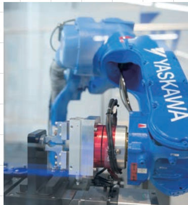
嵌合・はめ合いロボット (CSプラザ)
