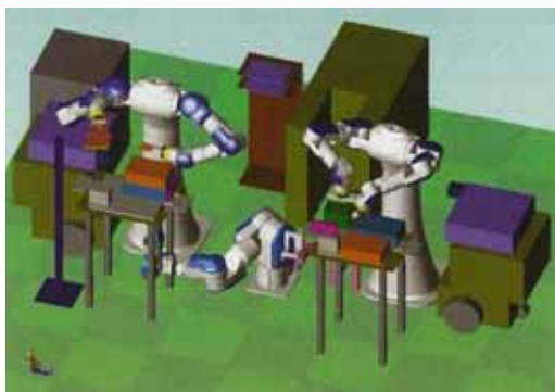
組立て・試験工程
