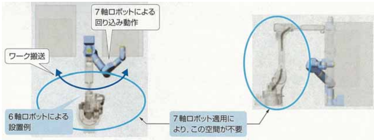
マシン間ハンドリング(回り込み姿勢)
