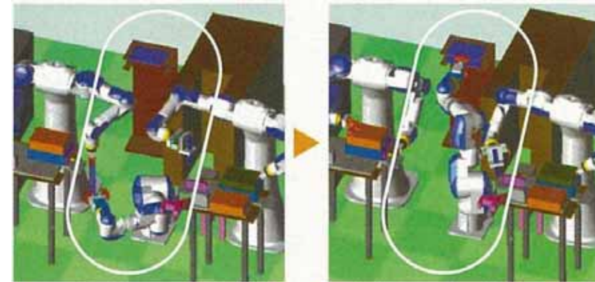
手前から奥へのワーク搬送を省スペースで実現
