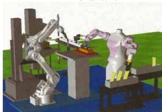
溶接工程における溶接ロボット との協調作業
